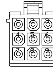
ENCODER 접속도
