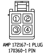
MOTOR CONNECTOR 접속도
