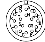
MS3102A20-29P Encoder Cable Connector 접속도
